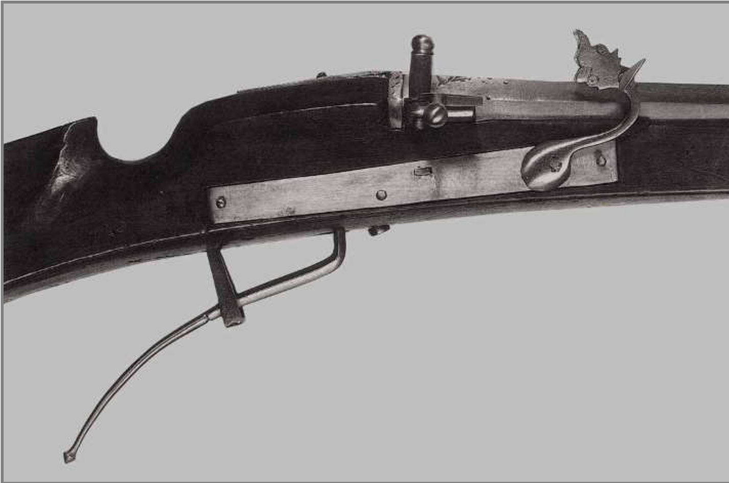
Luntenschloss der Muskete, um 1570
